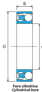
Foro cilindrico Cylindrical bore
