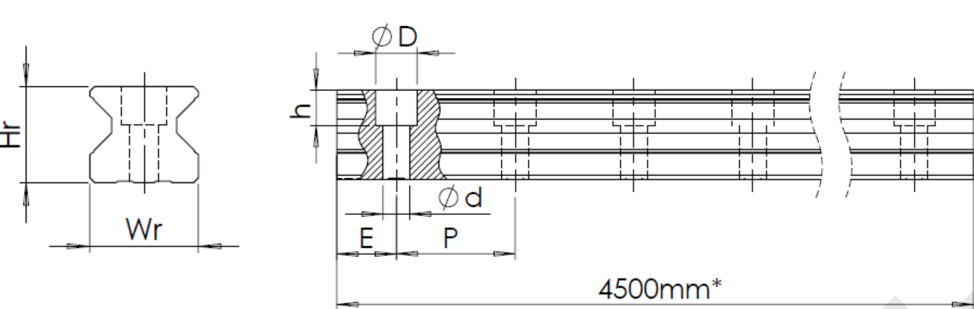
Роликовая направляющая стандартной длины BR-RGR R 25-55
