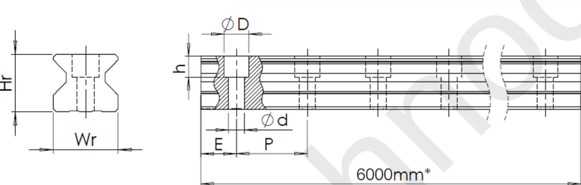
Роликовая направляющая стандартной длины BR-RGR R 65
