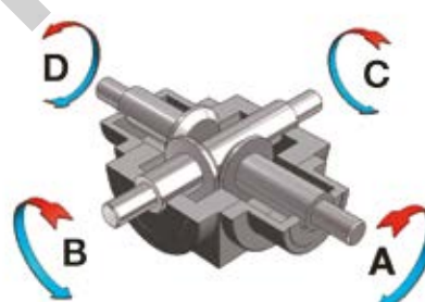
TIPO • TYPE 6
