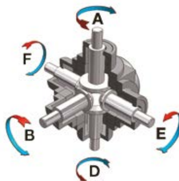
TIPO • TYPE 54
