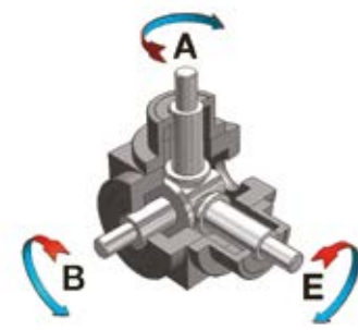
TIPO • TYPE 41
