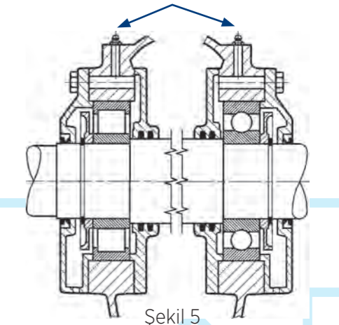
Ön Makaralı rulman Arka Sabitlenmiş yatak Şekil 5
