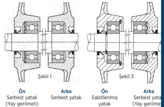
Ön Serbest yatak (Yay gerilmeli) Arka Serbest yatak (Yay gerilmeli) Ön Sabitlenmiş yatak Arka Serbest yatak (Yay gerilmeli)
