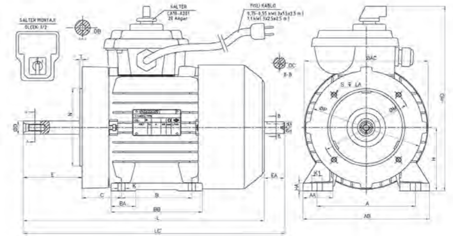
Ayaklı motor boyutları: B3, B6, B7, B8, B15, V5, V6 yapı biçimlerinde
