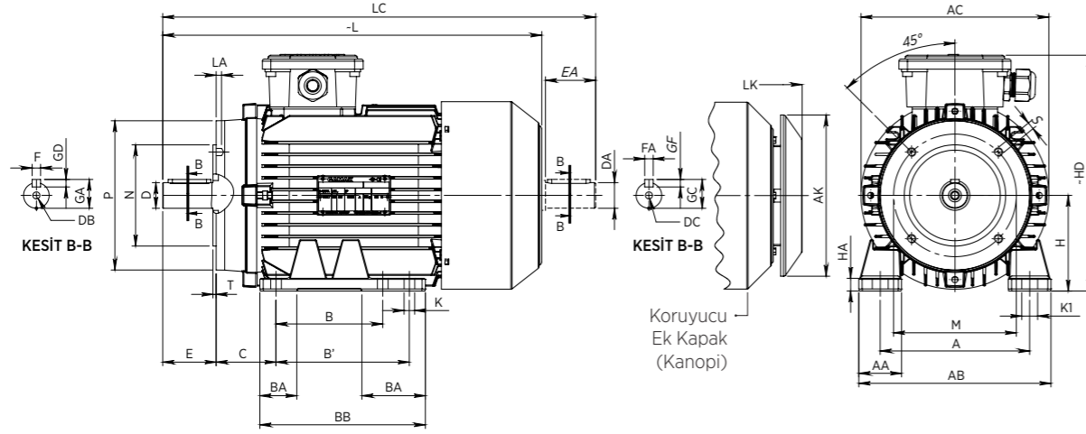
Ayaklı ve flanşlı motor boyutları: (Flanş biçimi C - DIN EN 50 347) B34 yapı biçiminde
