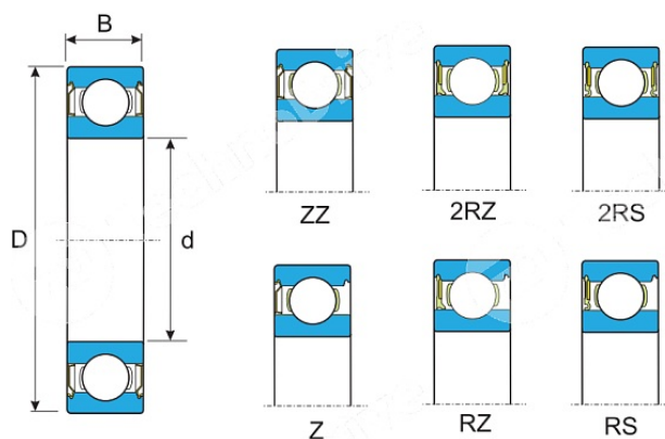
Внутренний диаметр - d Внешний диаметр - D Ширина подшипника B - B
