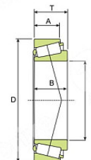
ОДНОРЯДНЫЕ КОНИЧЕСКИЕ РОЛИКОПОДШИПНИКИ (метрическая серия)
